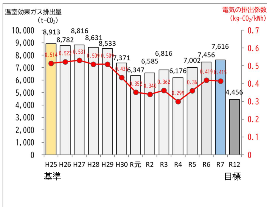
温室効果ガス排出量の推移
