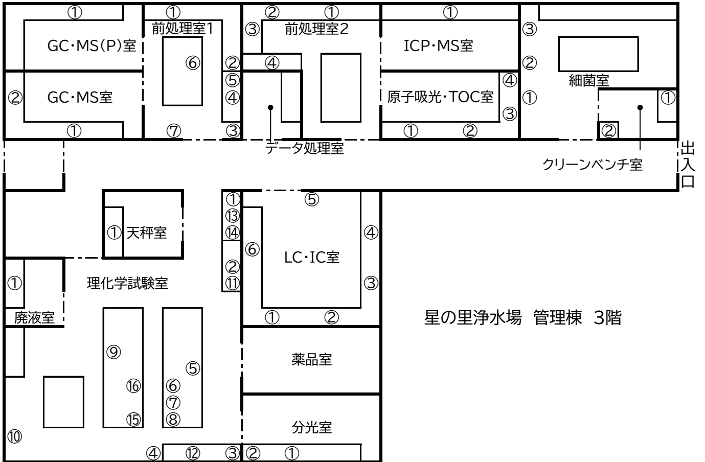
水質試験室平面図
