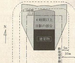
5階建マンションの日影（第2種住居専用地域、第2種高度地区の場合）
