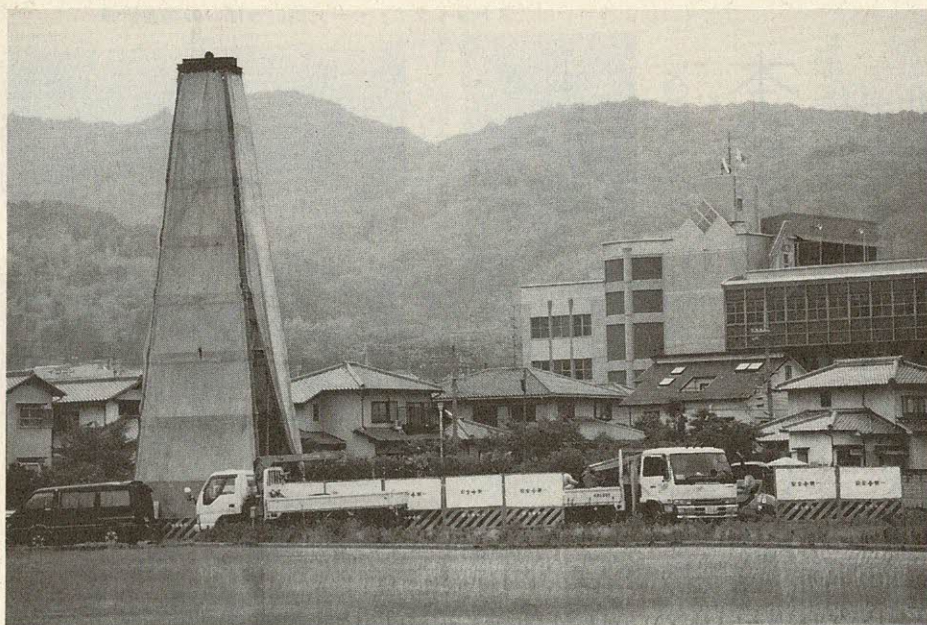
水確保のための掘り替え工事 (天野が原町)
