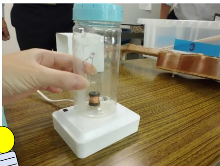
コイルを近づけると発電します。
