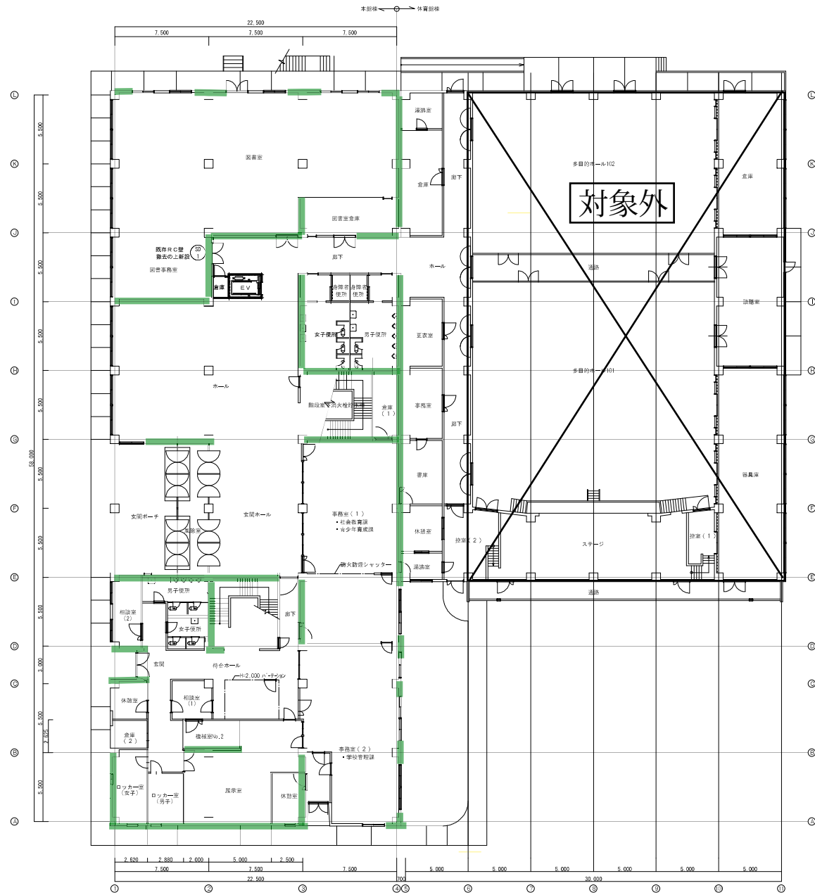
1階平面図 1/150
