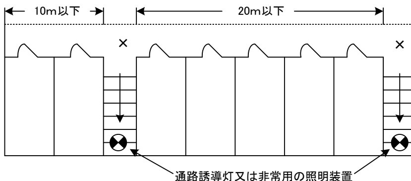
避難口誘導灯の設置に関し特例を適用できる場合
