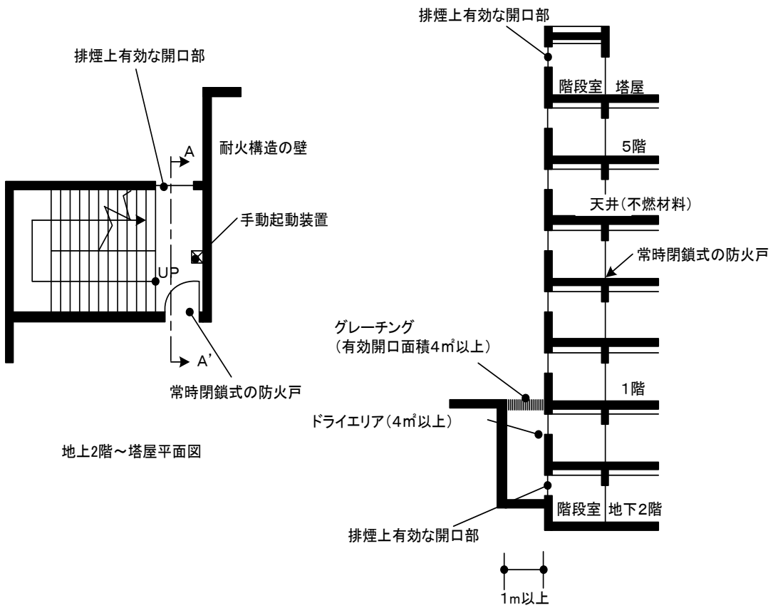
A～A' 断面図
