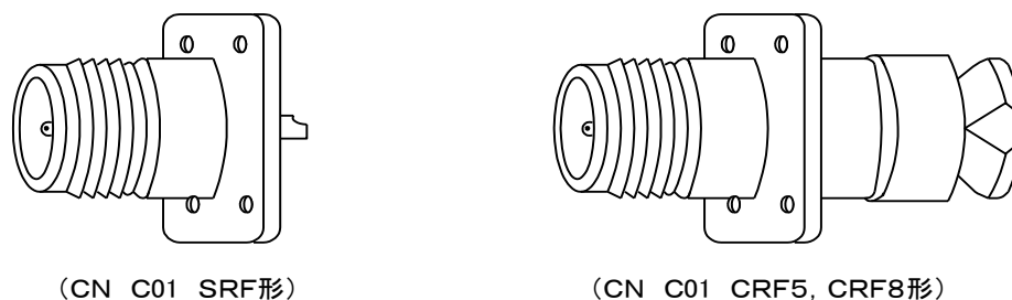
J I S C 5411C01形コネクタ外観図
