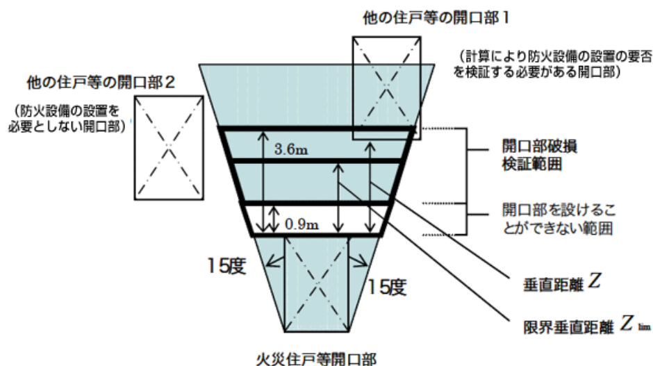
火災住戸等の開口部から噴出する火炎の影響を考慮すべき範囲
